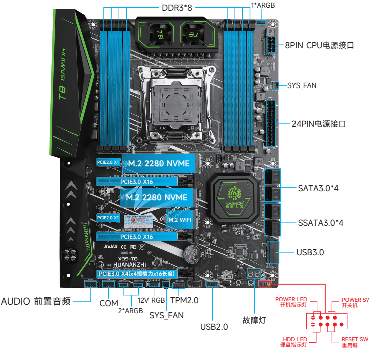
图1-1 X99-T8主板图解
